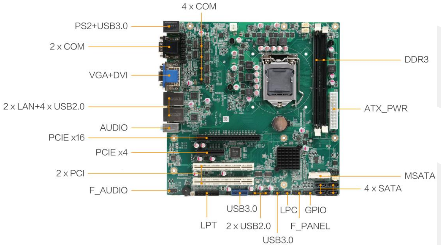
接口位置图
